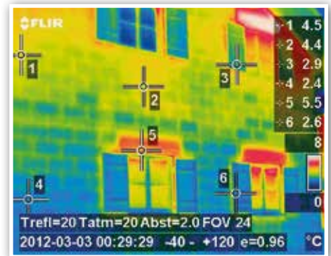
schlecht isolierte Fensterstürze/ ungedämmte Außenfassade sichtbar
