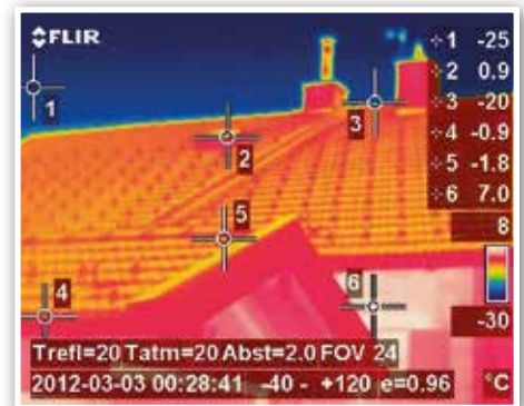
schlecht isoliertes Dach (hoher Wärmeübertrag über ganze Fläche)
